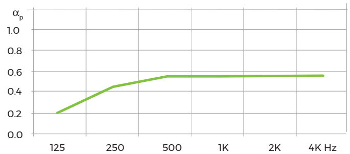
Plenum de 63
