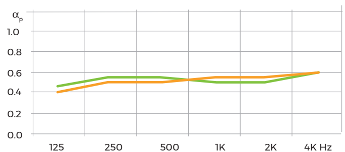
Plenum de 200 (1)
