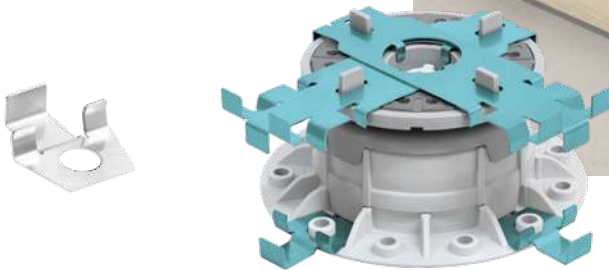
Pieza Inferior Bottom Piece
